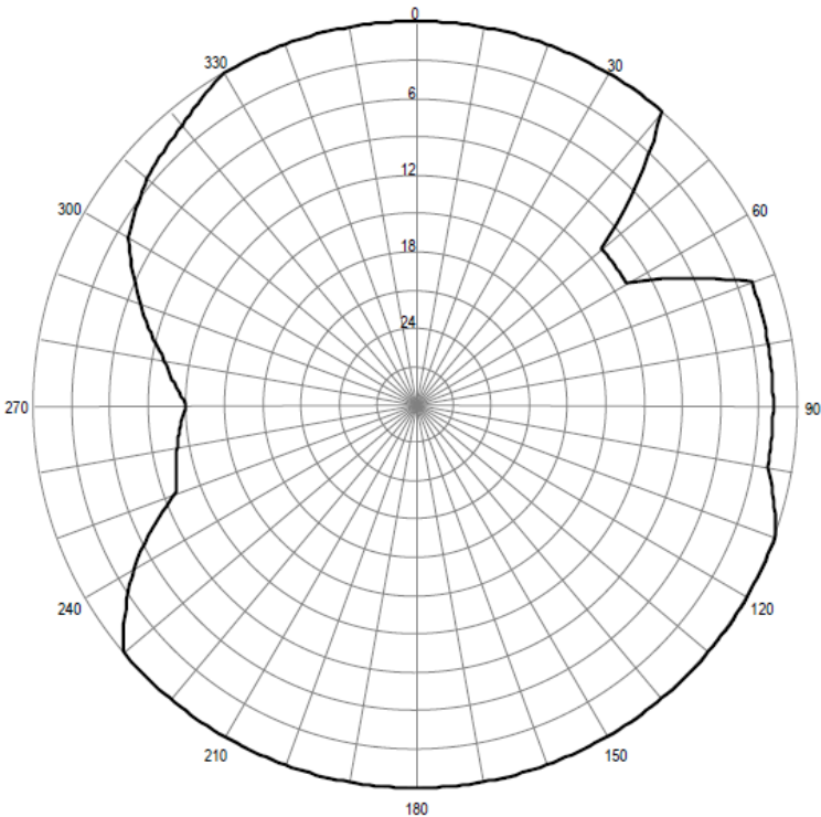
Pozioma charakterystyka promieniowania anteny stacji Wejherowo 88,00 MHz
