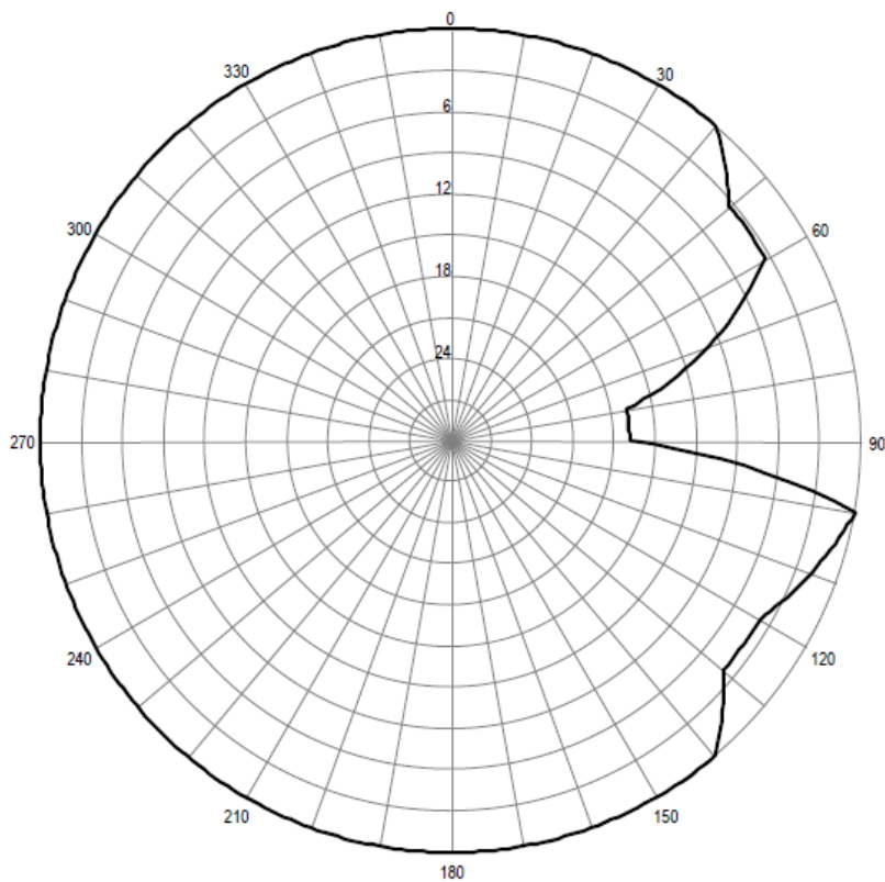
Pozioma charakterystyka promieniowania anteny stacji Reda 93,60 MHz
