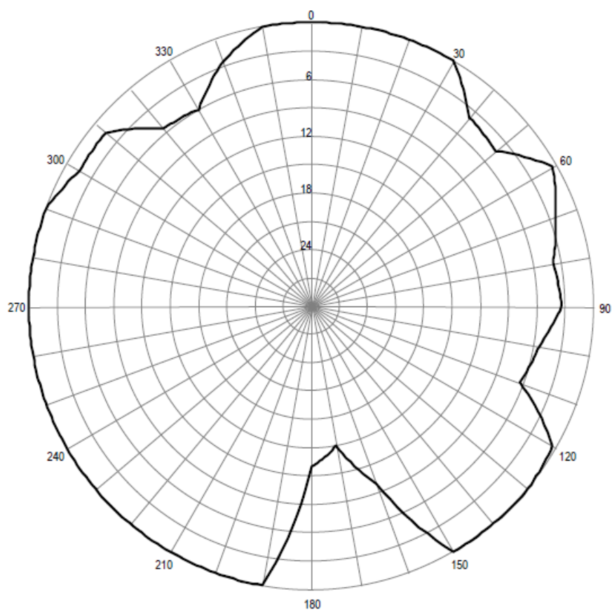
Pozioma charakterystyka promieniowania anteny stacji Gorzów Wielkopolski 101,70 MHz
