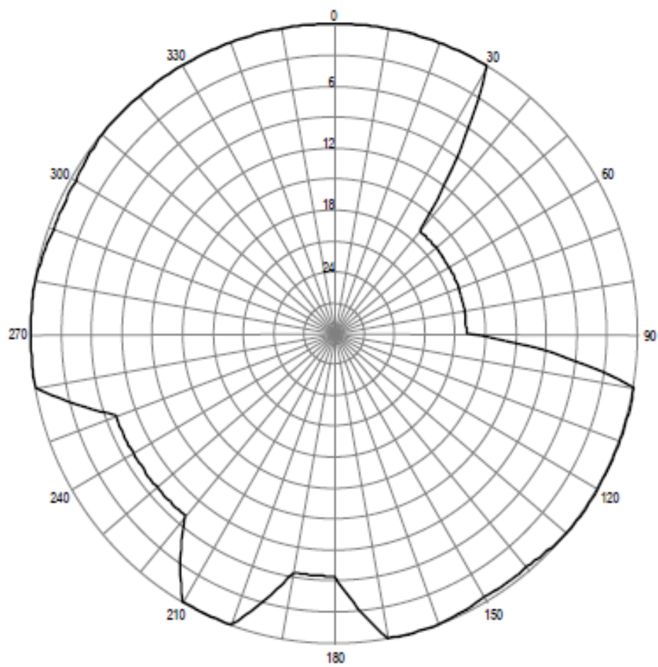
Pozioma charakterystyka promieniowania anteny stacji Gdańsk 90,0 MHz
