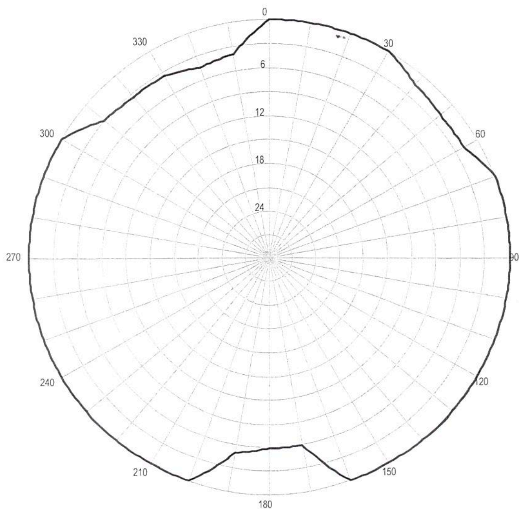
Pozioma charakterystyka promieniowania anteny stacji Ostrzeszów 96,90 MHz
