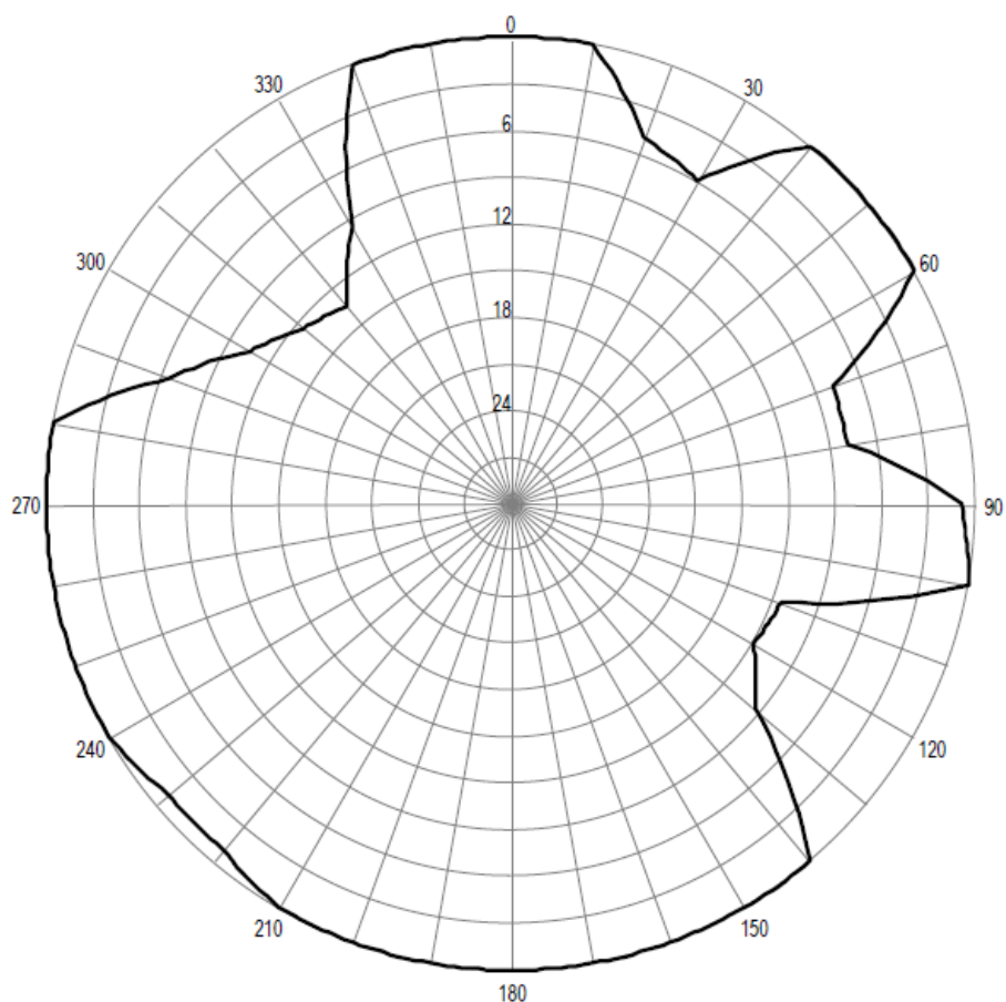
Pozioma charakterystyka promieniowania anteny stacji Zaniemyśl 95,20 MHz
