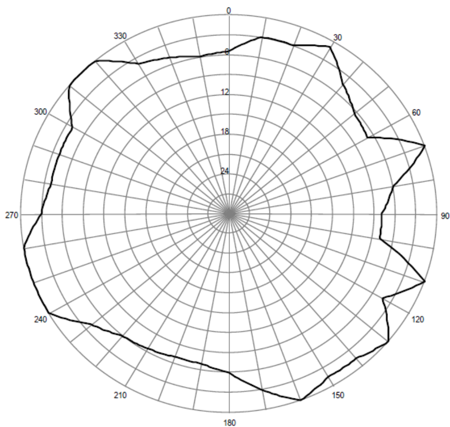
Pozioma charakterystyka promieniowania anteny stacji Września 93,70 MHz
