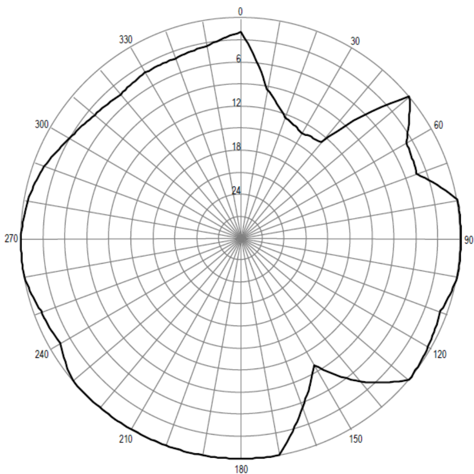
Pozioma charakterystyka promieniowania anteny stacji Topola Mała 94,90 MHz
