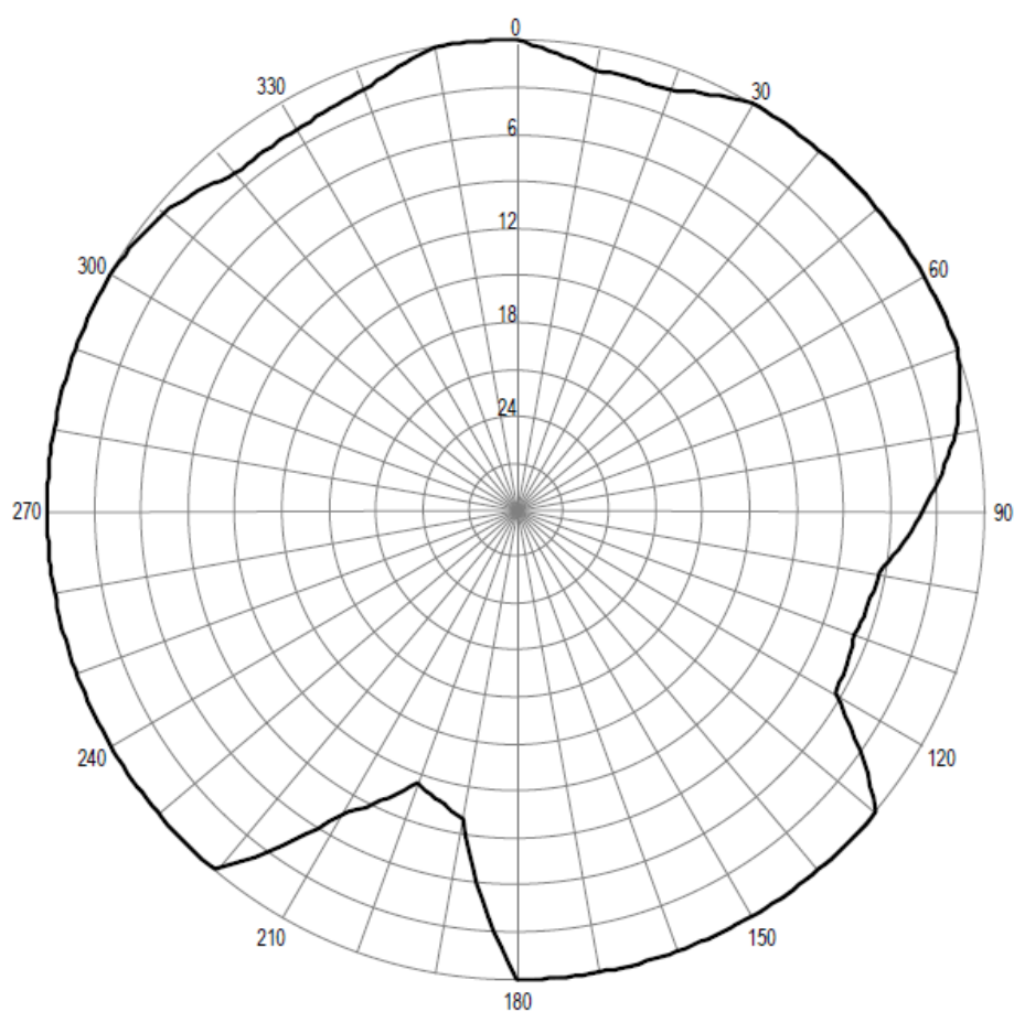
Pozioma charakterystyka promieniowania anteny stacji Jarocin 103,70 MHz
