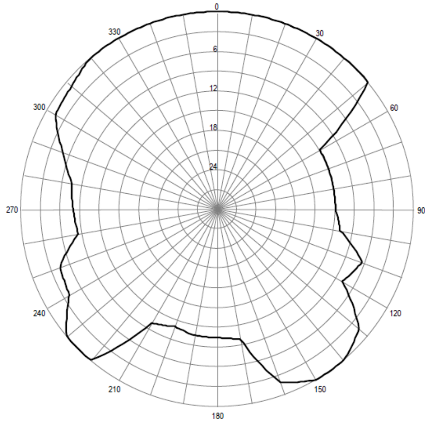
Pozioma charakterystyka promieniowania anteny stacji Inowrocław 98,10 MHz
