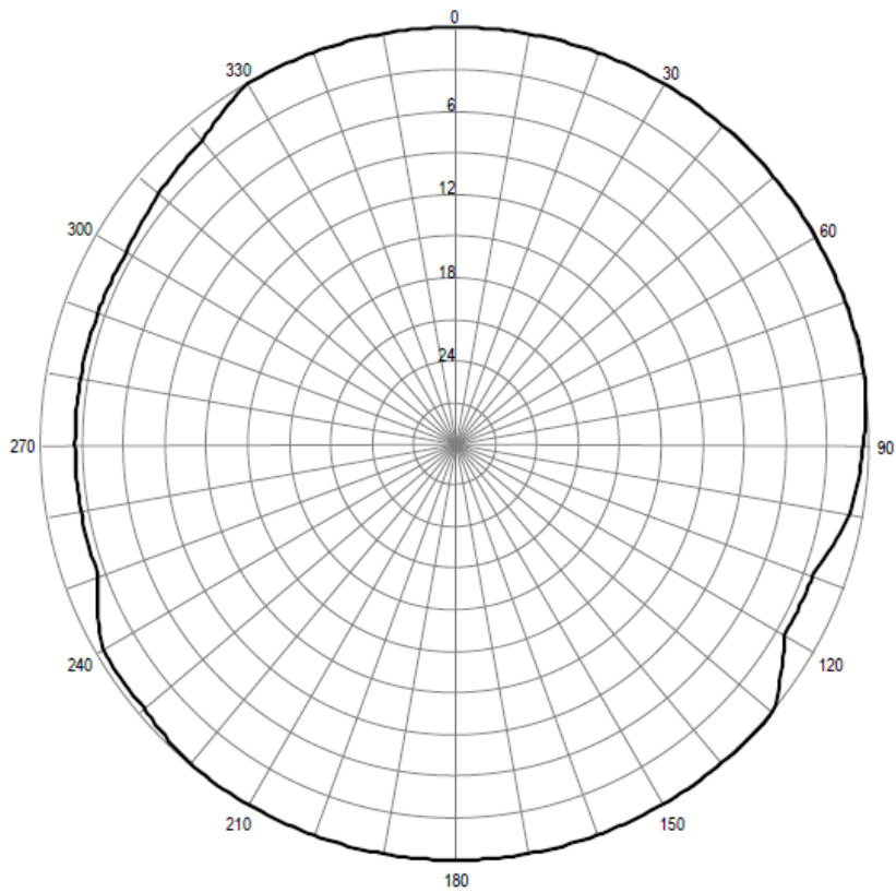
Pozioma charakterystyka promieniowania anteny stacji Siemianowice Śląskie 93,60 MHz
