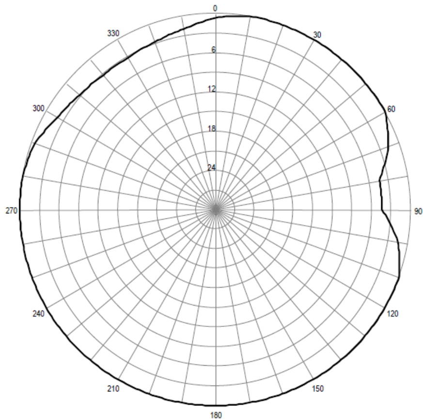
Pozioma charakterystyka promieniowania anteny stacji Grodzisk Mazowiecki 94,50 MHz
