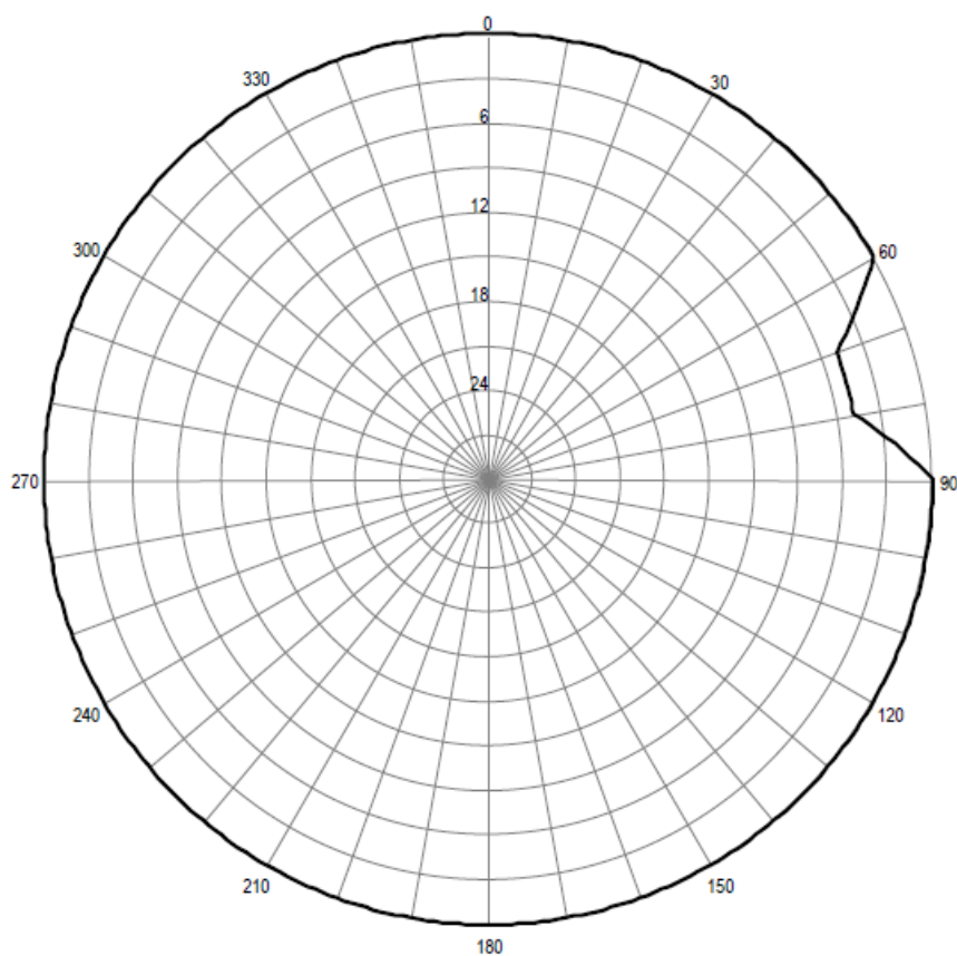
Pozioma charakterystyka promieniowania anteny stacji Żyrardów 104,10 MHz
