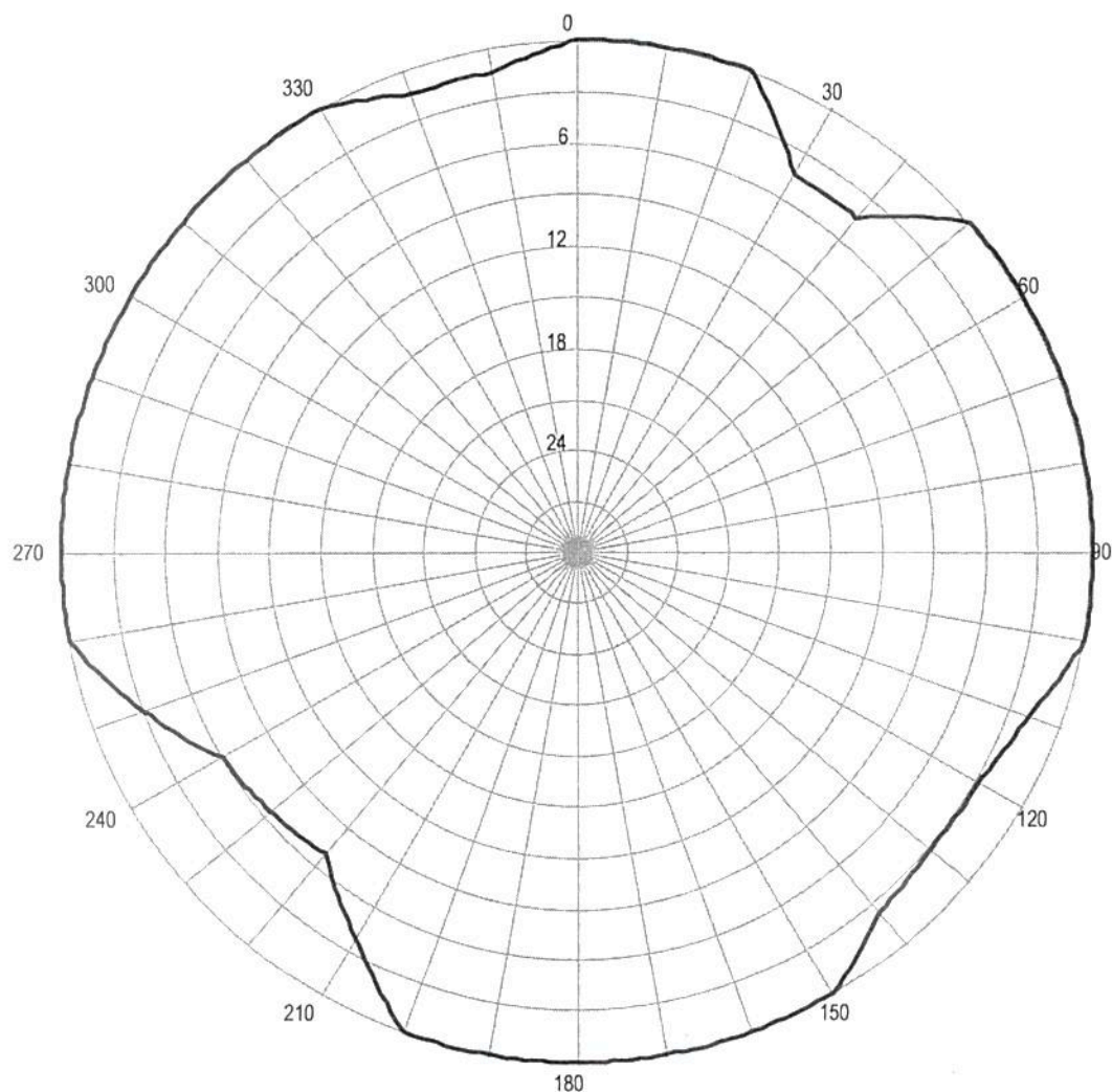
Pozioma charakterystyka promieniowania anteny stacji Tarnów G. Św. Marcina 92,8 MHz
