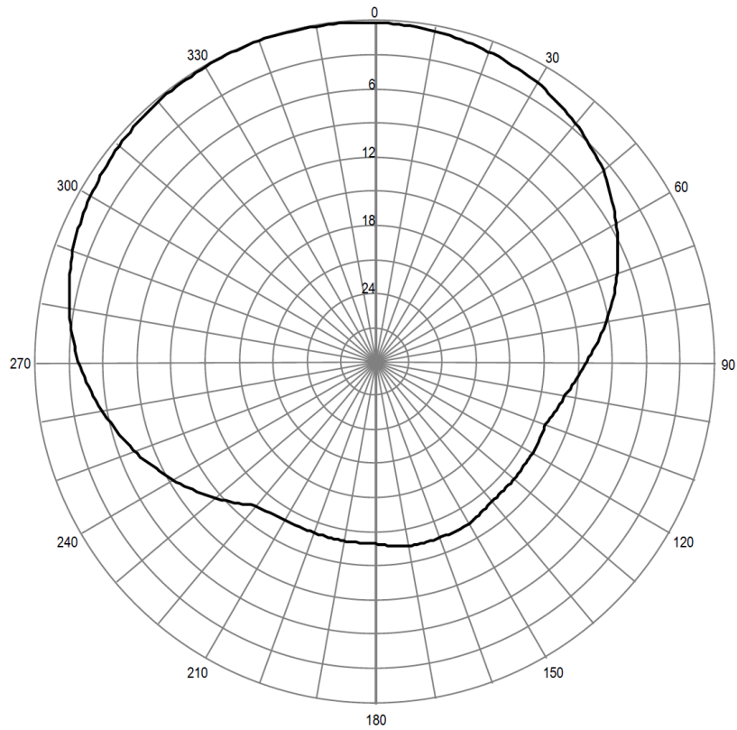
Pozioma charakterystyka promieniowania anteny stacji Góra Bełchówka k/ Bukowska 95,20 MHz
