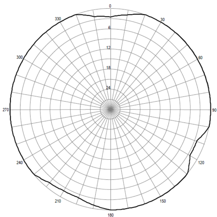
Pozioma charakterystyka promieniowania anteny stacji Naklo n. Notecią 107,50 MHz
