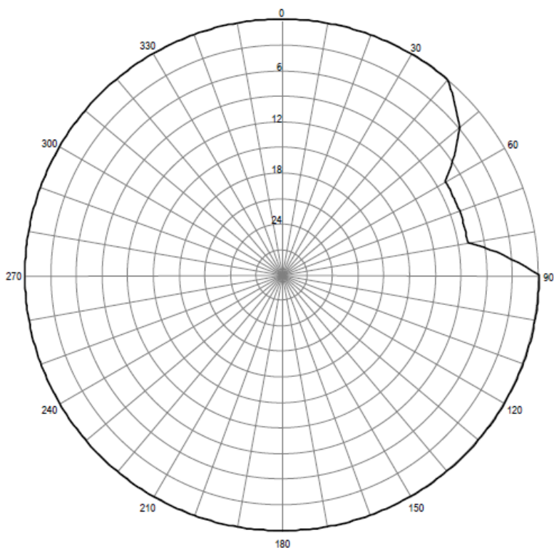
Pozioma charakterystyka promieniowania anteny stacji Gdańsk 103,0 MHz
