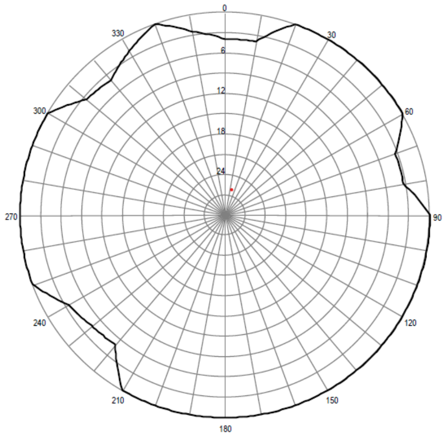
Pozioma charakterystyka promieniowania anteny stacji Grudziądz 90,60 MHz
