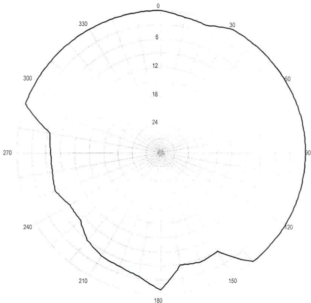
Pozioma charakterystyka promieniowania anteny stacji Jędrzejów 93,2 MHz
