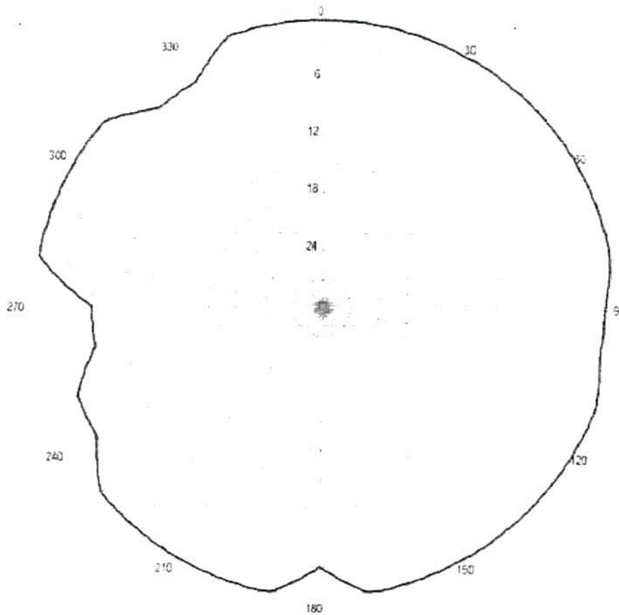
Pozioma charakterystyka promieniowania anteny stacji Puławy 97,2 MHz
