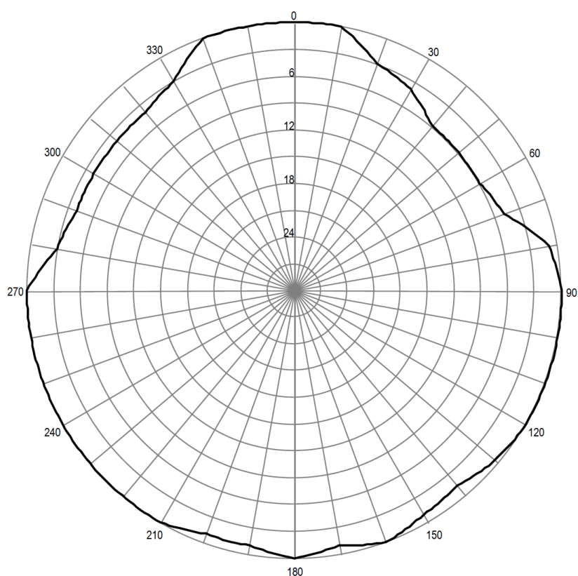
Pozioma charakterystyka promieniowania anteny stacji Warszawa 100,10 MHz
