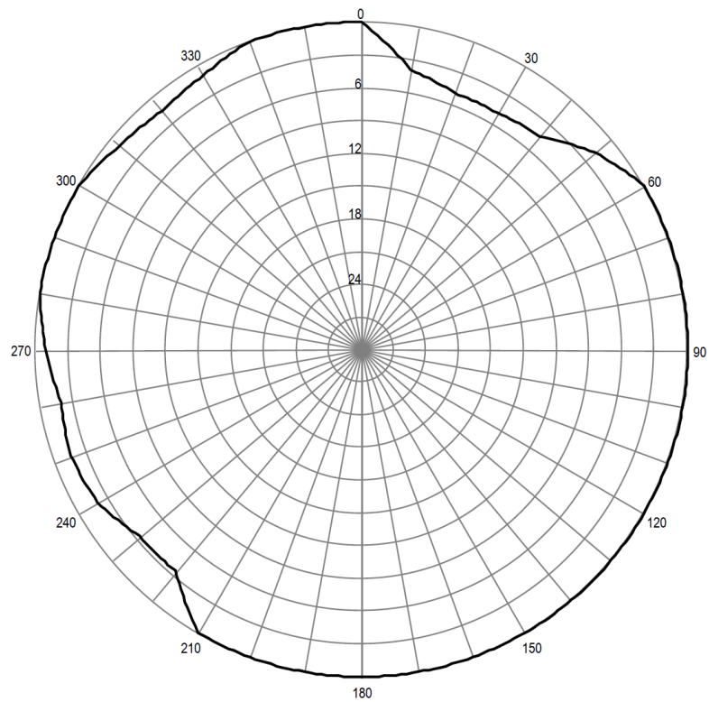
Pozioma charakterystyka promieniowania anteny stacji Warszawa 103,70 MHz
