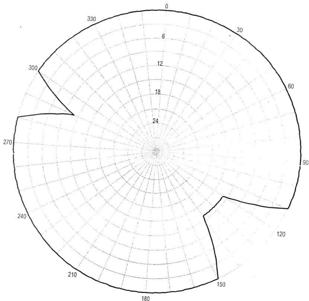
Pozioma charakterystyka promieniowania anteny stacji Sanok 95,20 MHz
