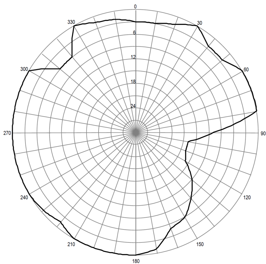
Pozioma charakterystyka promieniowania anteny stacji Pabianice 101,30 MHz
