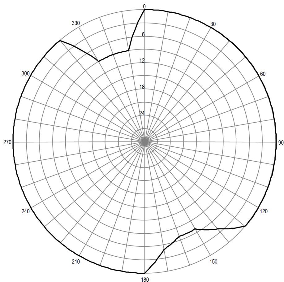
Pozioma charakterystyka promieniowania anteny stacji Łódź 88,80 MHz
