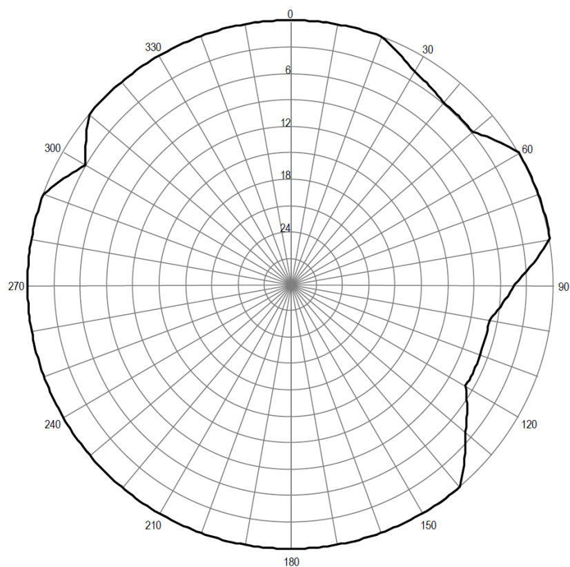
Pozioma charakterystyka promieniowania anteny stacji Włocławek 107,60 MHz
