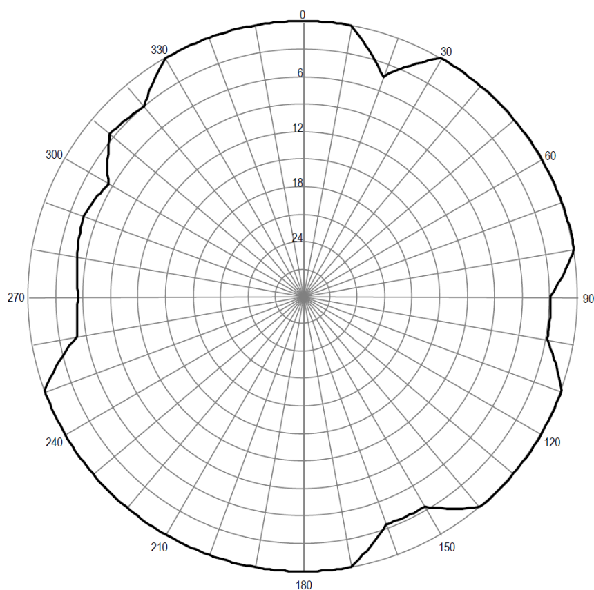
Pozioma charakterystyka promieniowania anteny stacji Morliny 101,50 MHz
