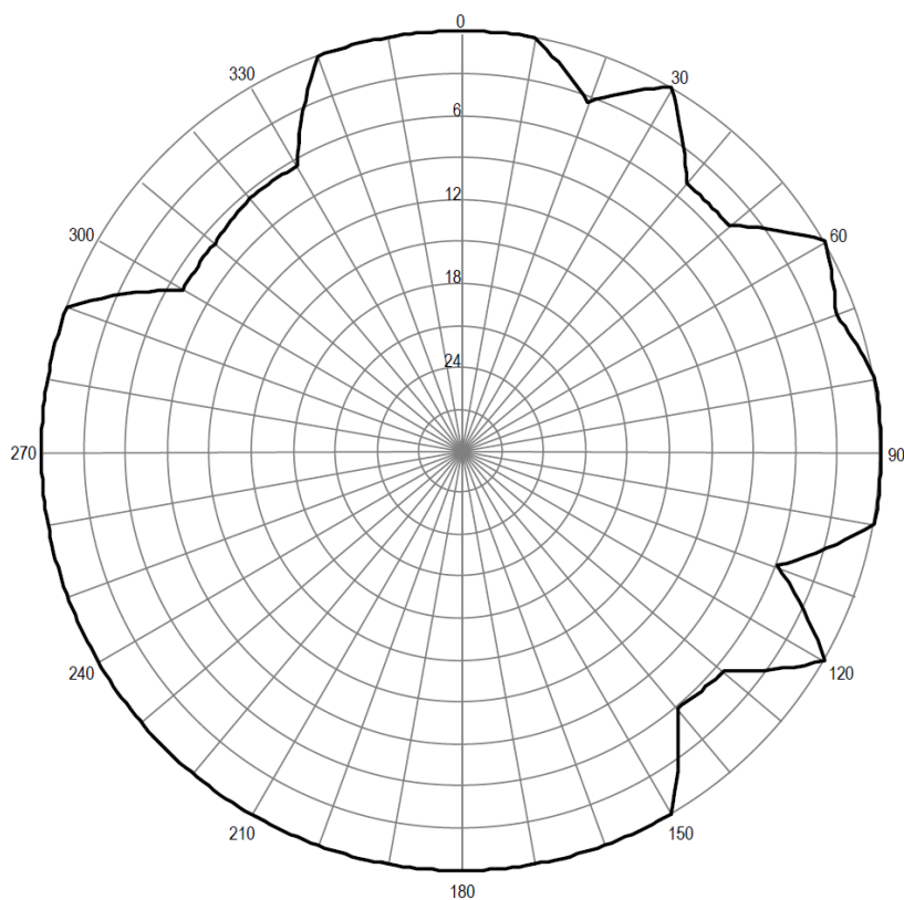
Pozioma charakterystyka promieniowania anteny stacji Olsztynek 89,40 MHz
