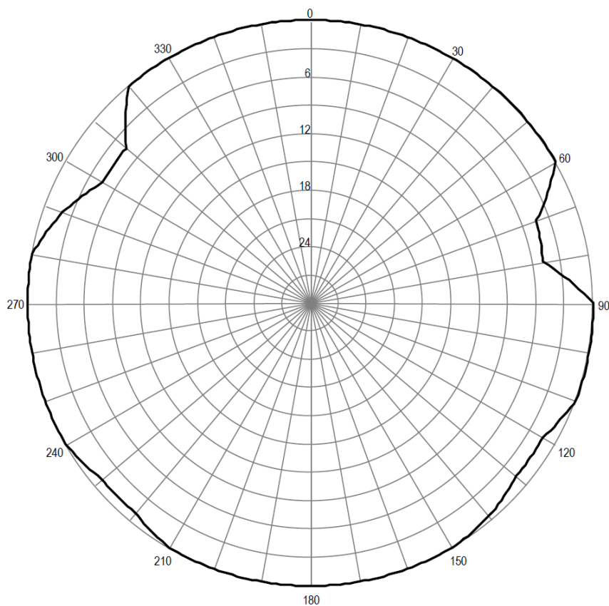
Pozioma charakterystyka promieniowania anteny stacji Morąg 96,40 MHz
