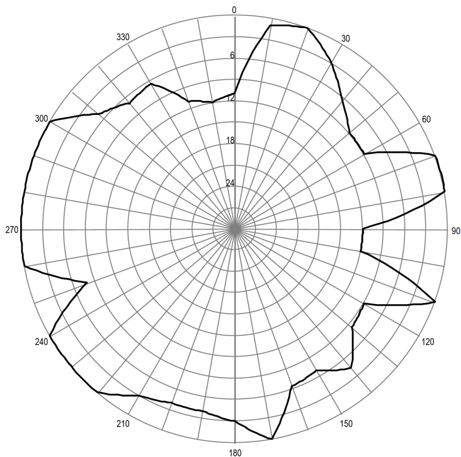
Pozioma charakterystyka promieniowania anteny stacji Zielona Góra 96,0 MHz
