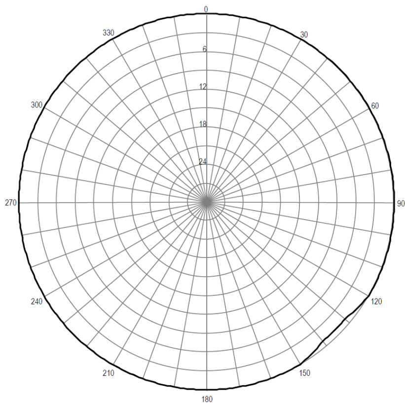
Pozzioma charakterystyka promieniowania anteny stacji Łysa Góra k/ Dziwiszowa 106,20 MHz
