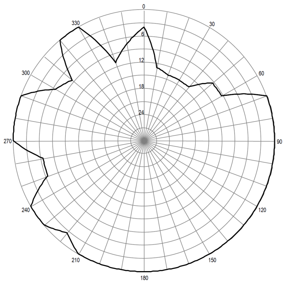
Pozioma charakterystyka promieniowania anteny stacji Opoczno 97,80 MHz
