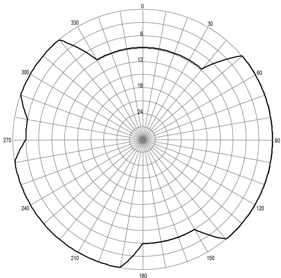
Pozioma charakterystyka promieniowania anteny stacji Łódź 96,0 MHz
