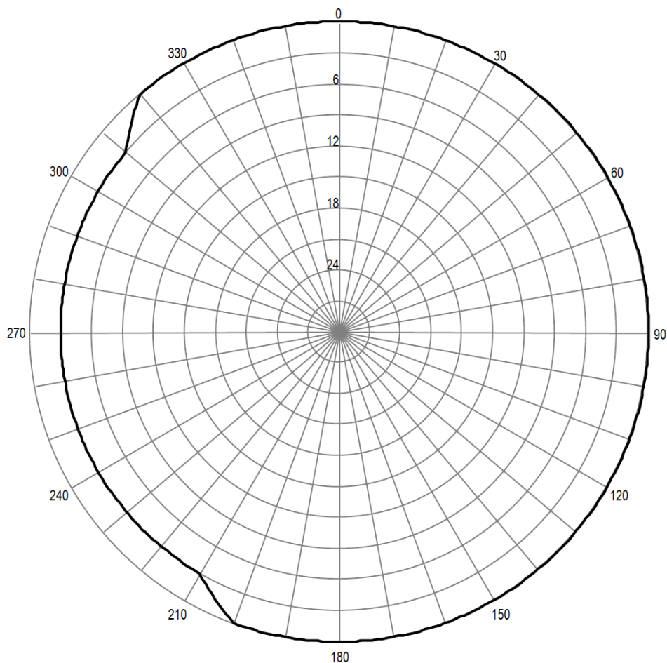
Pozioma charakterystyka promieniowania anteny stacji Wałbrzych 91,80 MHz
