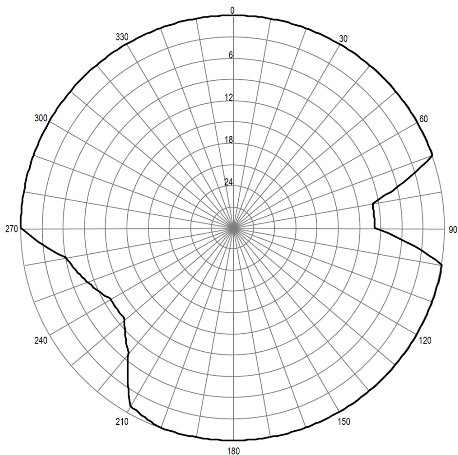
Pozioma charakterystyka promieniowania anteny stacji Białystok 101,0 MHz
