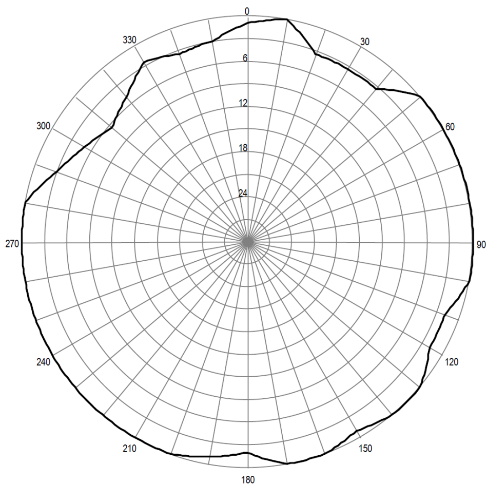
Pozioma charakterystyka promieniowania anteny stacji Kielce 103,90 MHz
