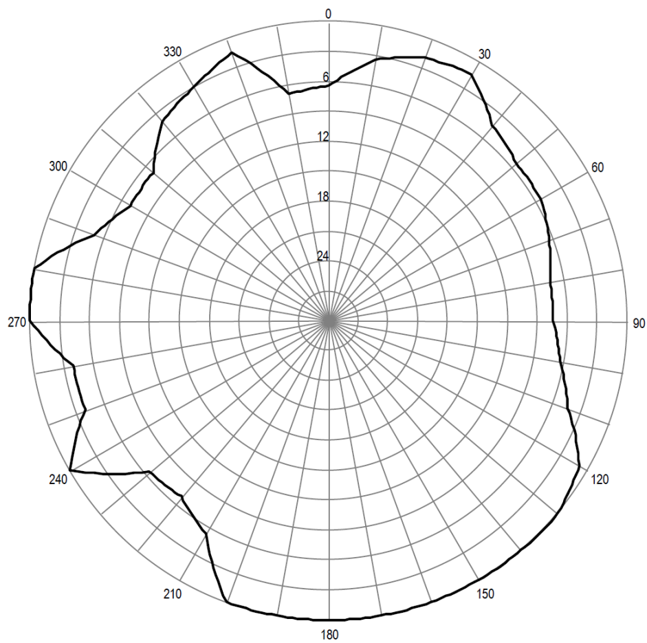
Pozioma charakterystyka promieniowania anteny stacji Dobromierz 101,10 MHz
