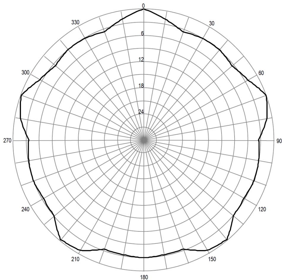
Pozioma charakterystyka promieniowania anteny stacji Kielce Św. Krzyż 106,50 MHz
