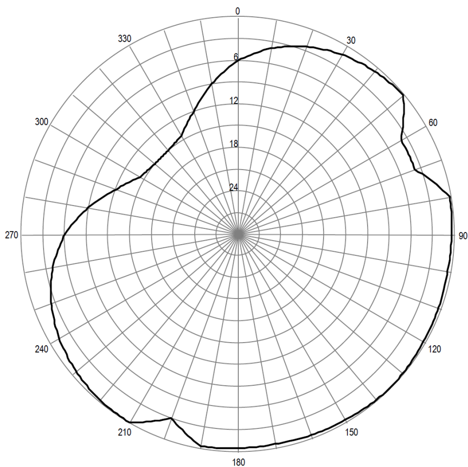
Pozioma charakterystyka promieniowania anteny stacji Szczecin Warszewo 89,80 MHz
