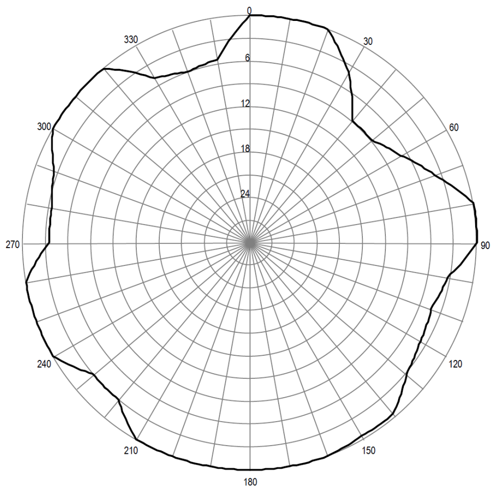
Pozioma charakterystyka promieniowania anteny stacji Bydgoszcz 90,50 MHz
