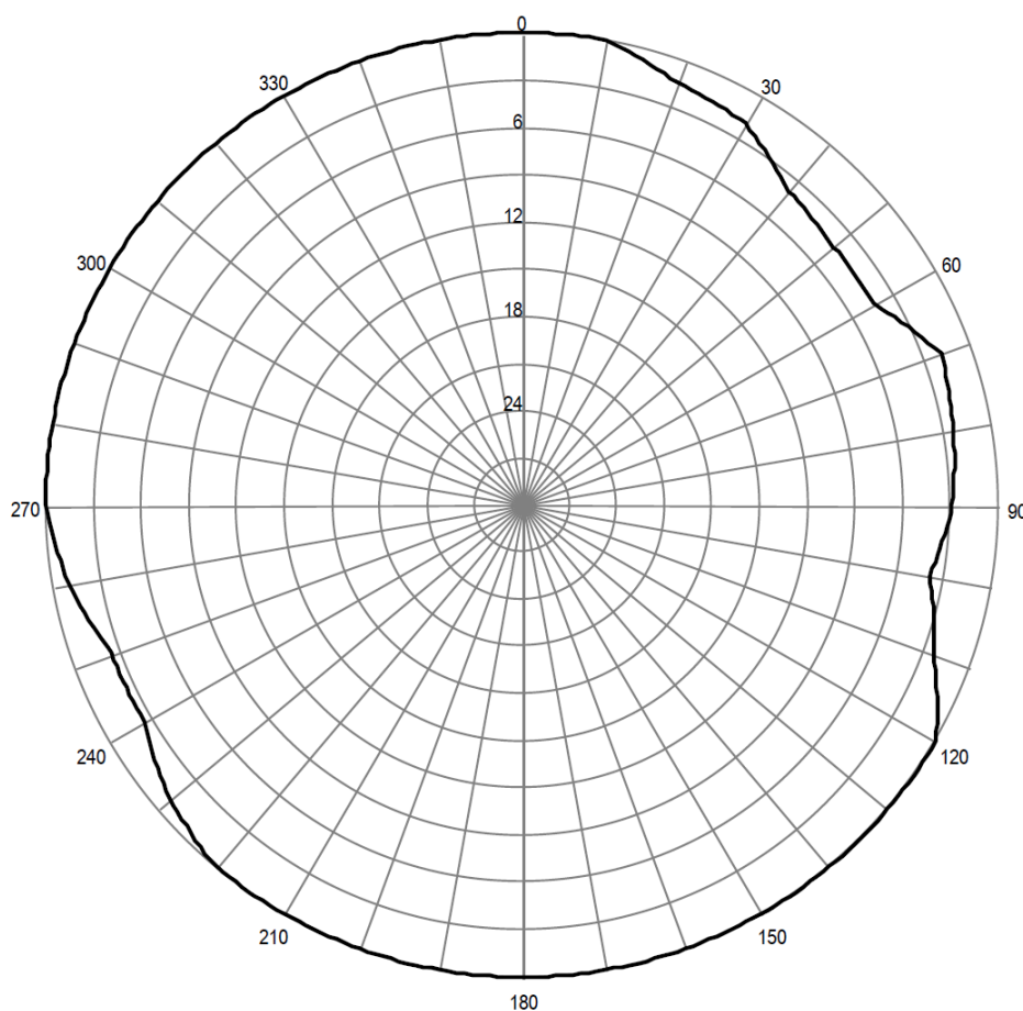
Pozioma charakterystyka promieniowania anteny stacji Łódź 102,30 MHz
