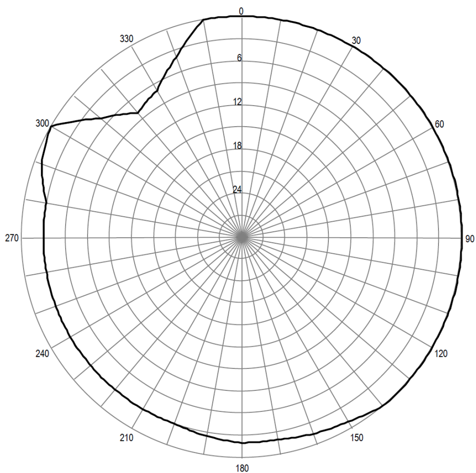
Pozioama charakterystyka promieniowania anteny stacji Kielce 92,90 MHz
