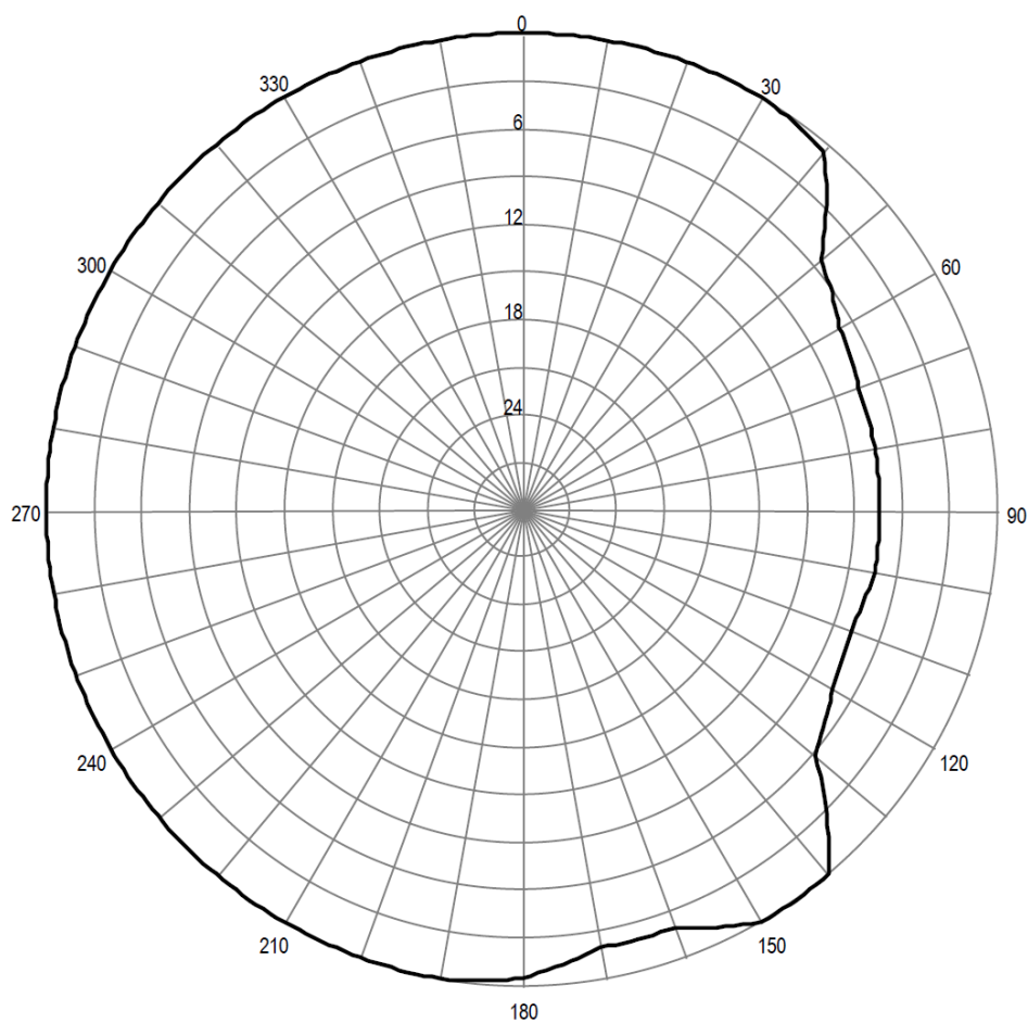
Pozioma charakterystyka promieniowania anteny stacji Olsztyn 92,40 MHz
