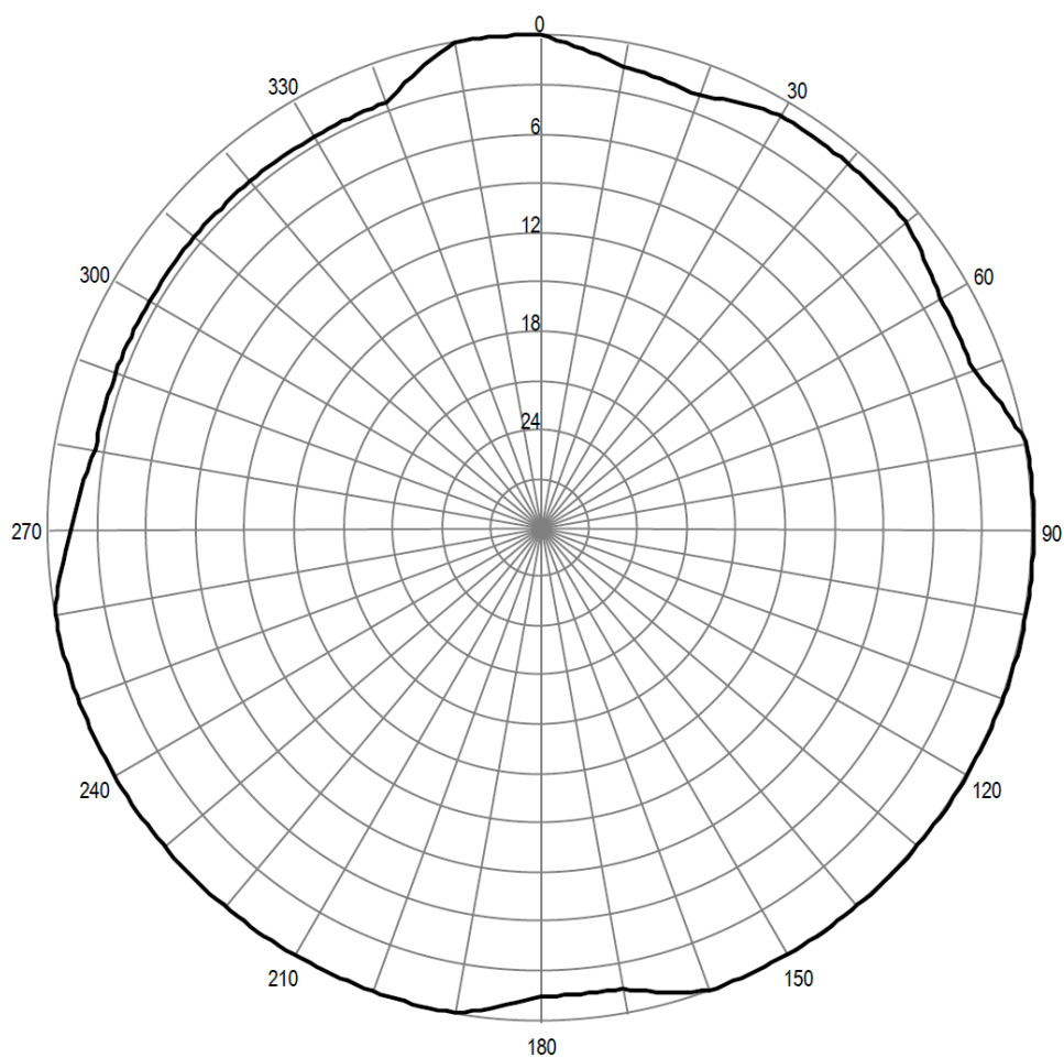
Pozioma charakterystyka promieniowania anteny stacji Warszawa 102,0 MHz
