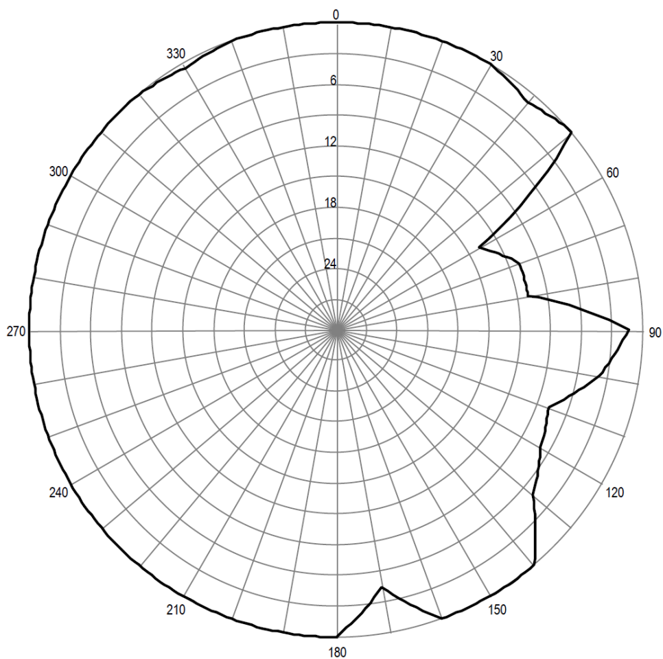
Pozioma charakterystyka promieniowania anteny stacji Gdańsk Jaśkowa Kopa 93,90 MHz
