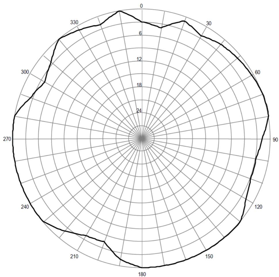
Pozioma charakterystyka promieniowania anteny stacji Warszawa 105,60 MHz
