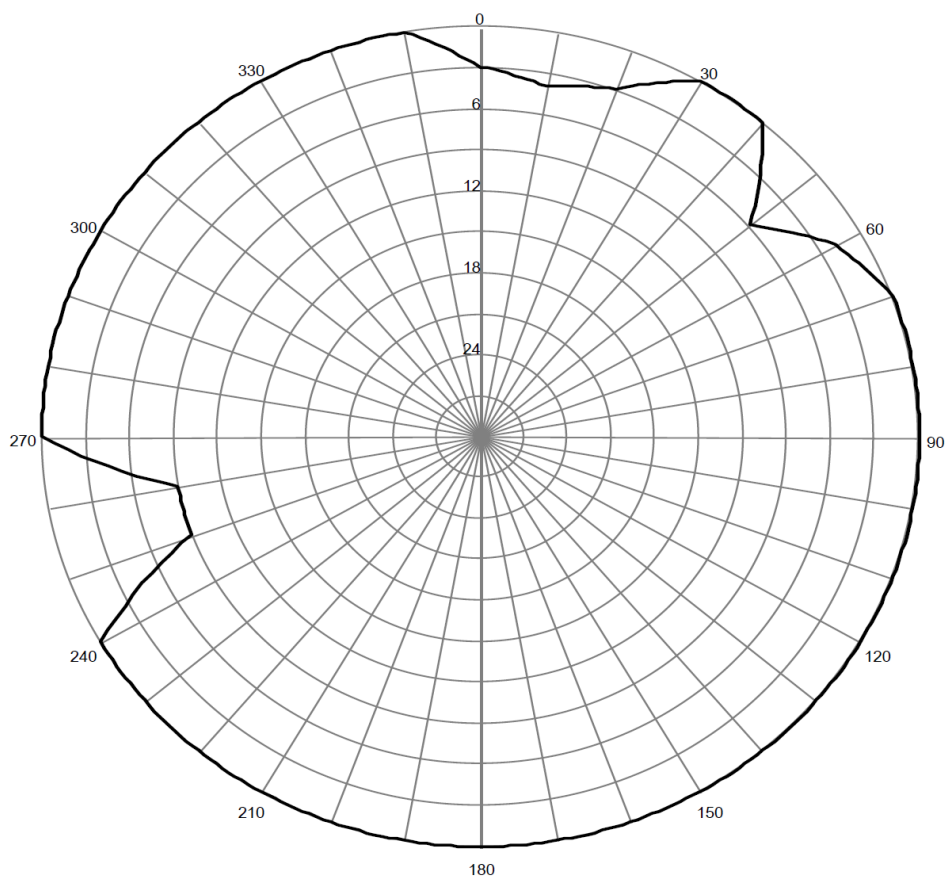
Pozioma charakterystyka promieniowania anteny stacji
