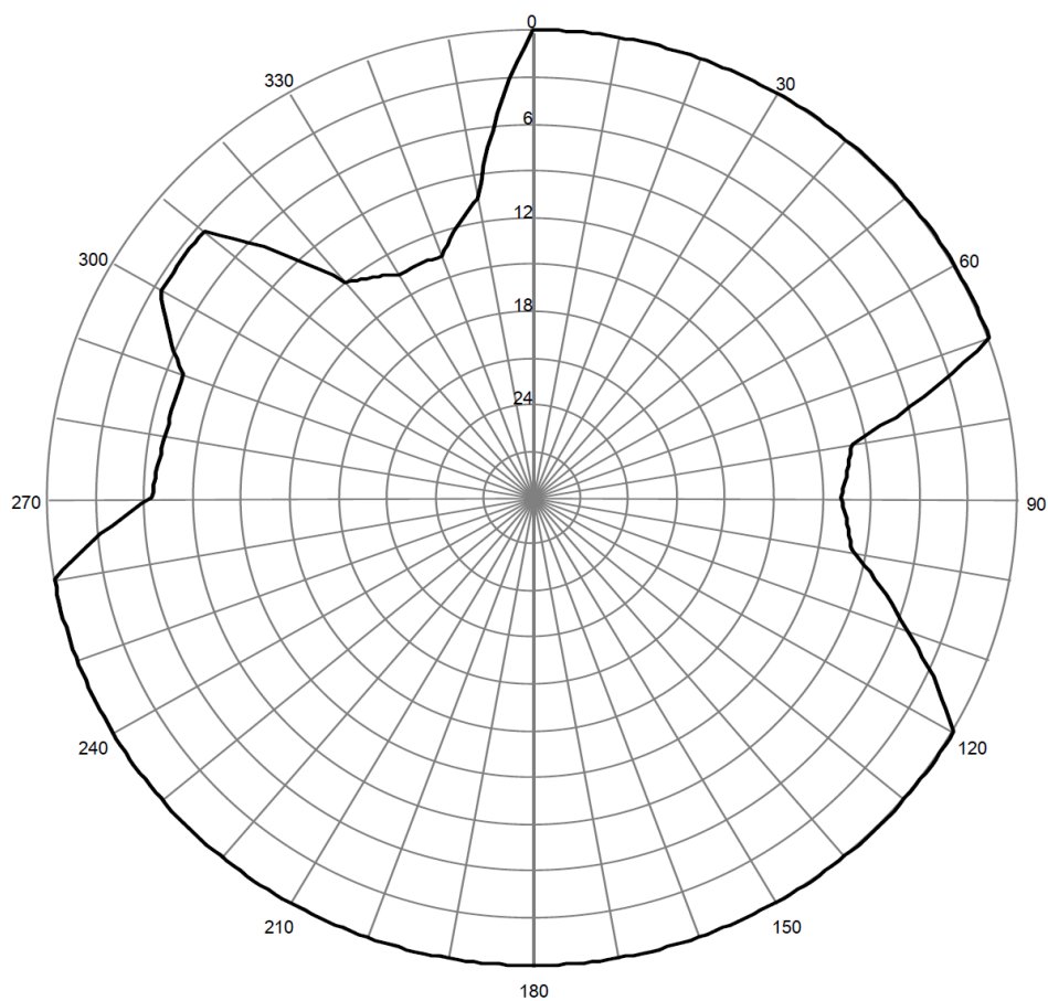
Pozioma charakterystyka promieniowania anteny stacji
