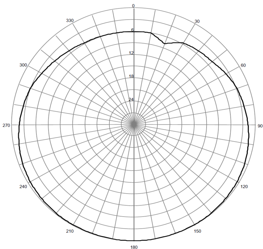
Pozioma charakterystyka promieniowania anteny stacji Kościerzyna 91,70 MHz
