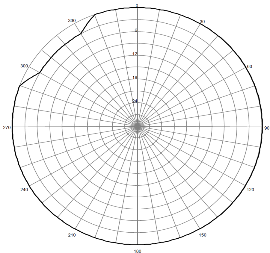
Pozioma charakterystyka promieniowania anteny stacji
