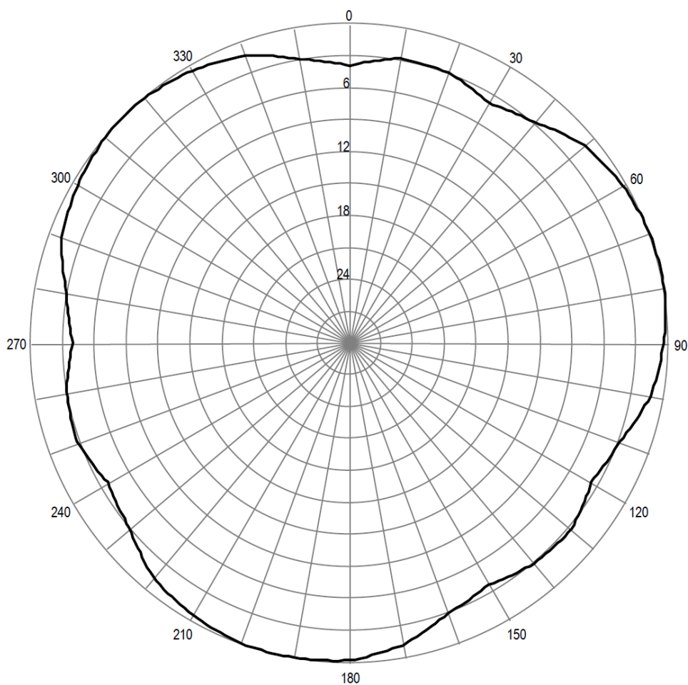
Pozioma charakterystyka promieniowania anteny stacji Poznań Śrem 106,20 MHz
