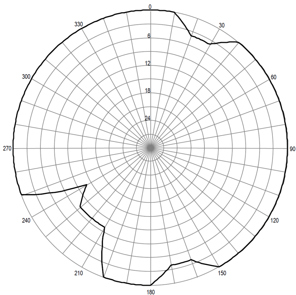
Pozioma charakterystyka promieniowania anteny stacji Bolewice 90,40 MHz
