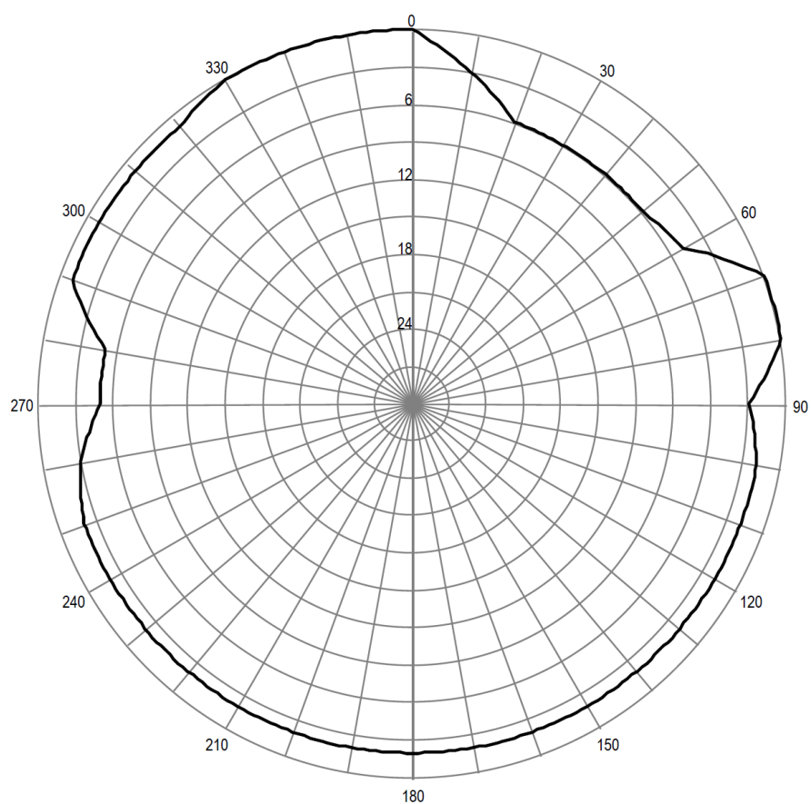
Pozioma charakterystyka promieniowania anteny stacji Gorzów Wielkopolski 93,80 MHz
