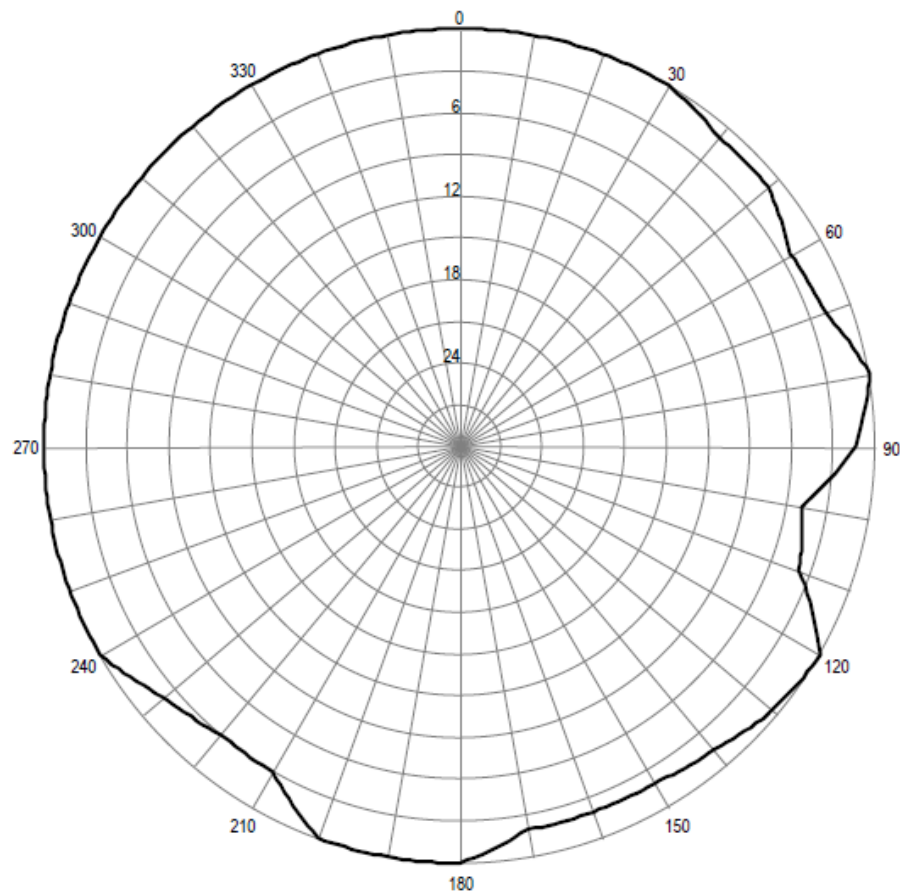
Pozioma charakterystyka promieniowania anteny stacji Szczecin Kołowo 88,90 MHz
