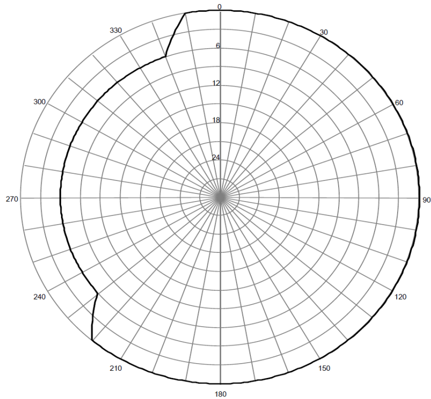
Pozioma charakterystyka promieniowania anteny stacji
