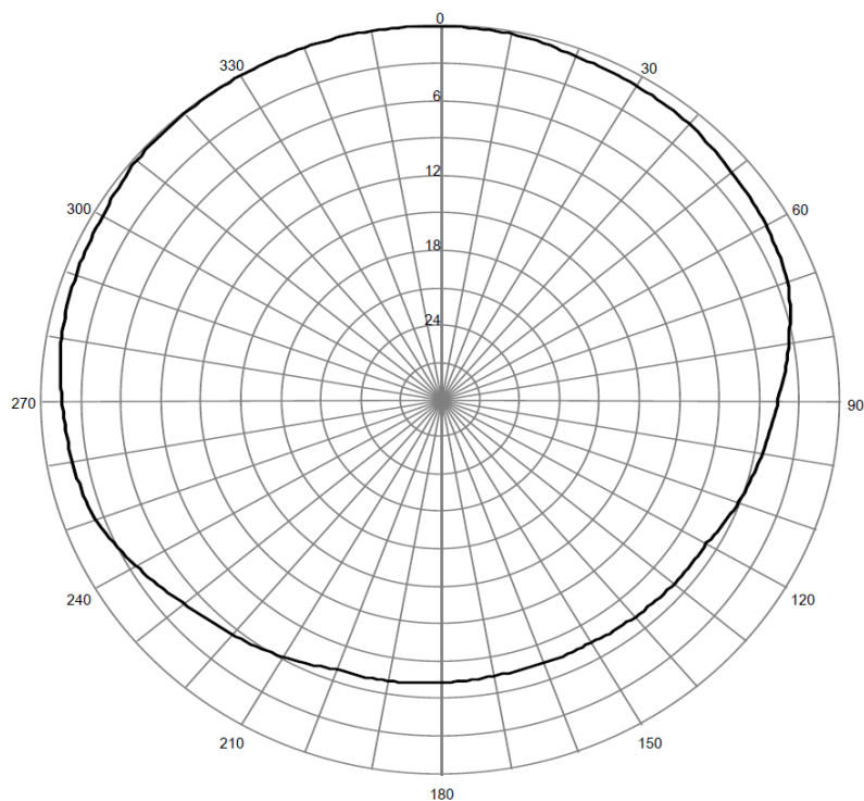
Pozioma charakterystyka promieniowania anteny stacji
