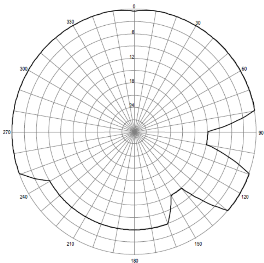
Pozioma charakterystyka promieniowania anteny stacji Góra Liwocz 94,10 MHz
