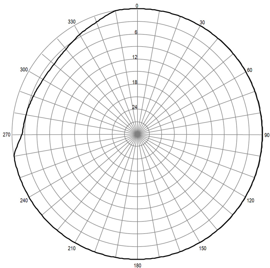
Pozioma charakterystyka promieniowania anteny stacji Radom 90,70 MHz
