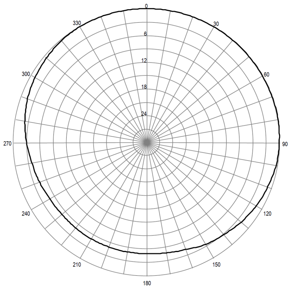
Pozioma charakterystyka promieniowania anteny stacji
