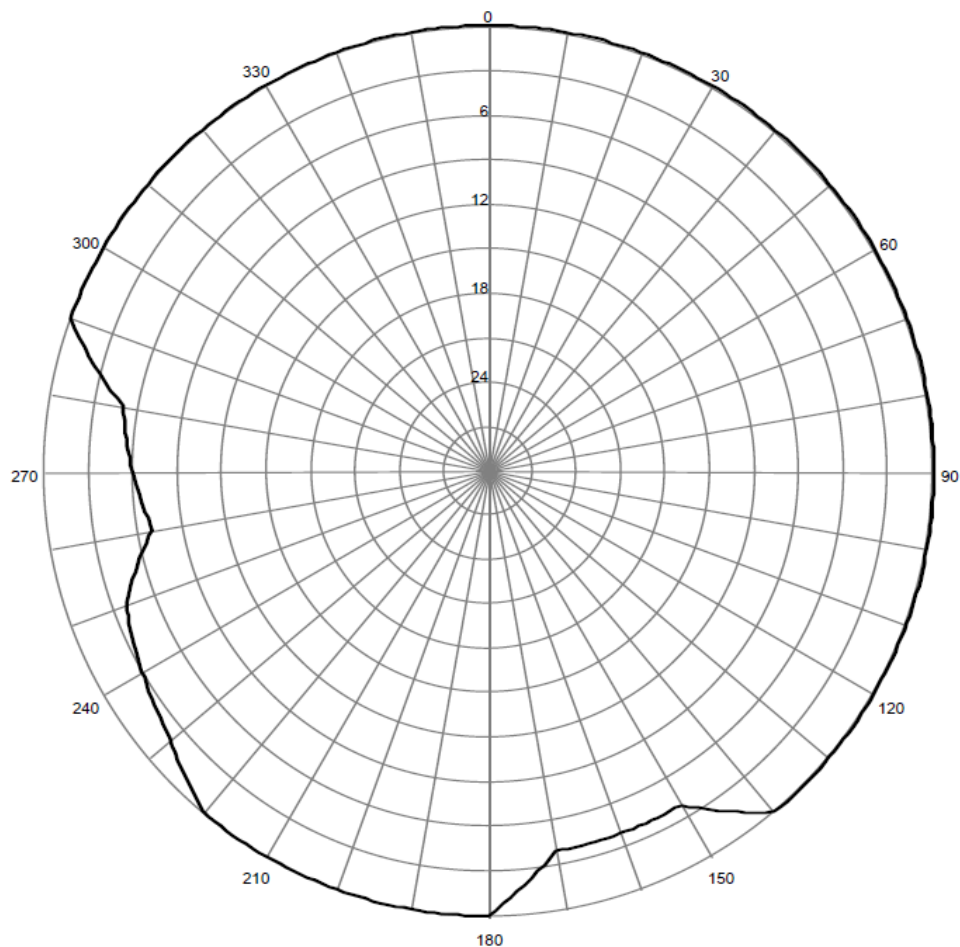
Pozioma charakterystyka promieniowania anteny stacji Leżajsk 93,0 MHz
