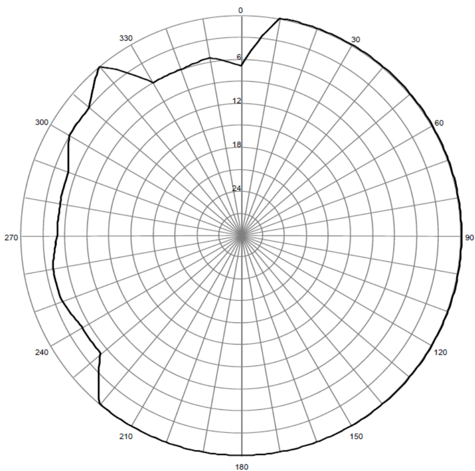
Pozioma charakterystyka promieniowania anteny stacji Średnia k/ Przemysła 98,20 MHz
