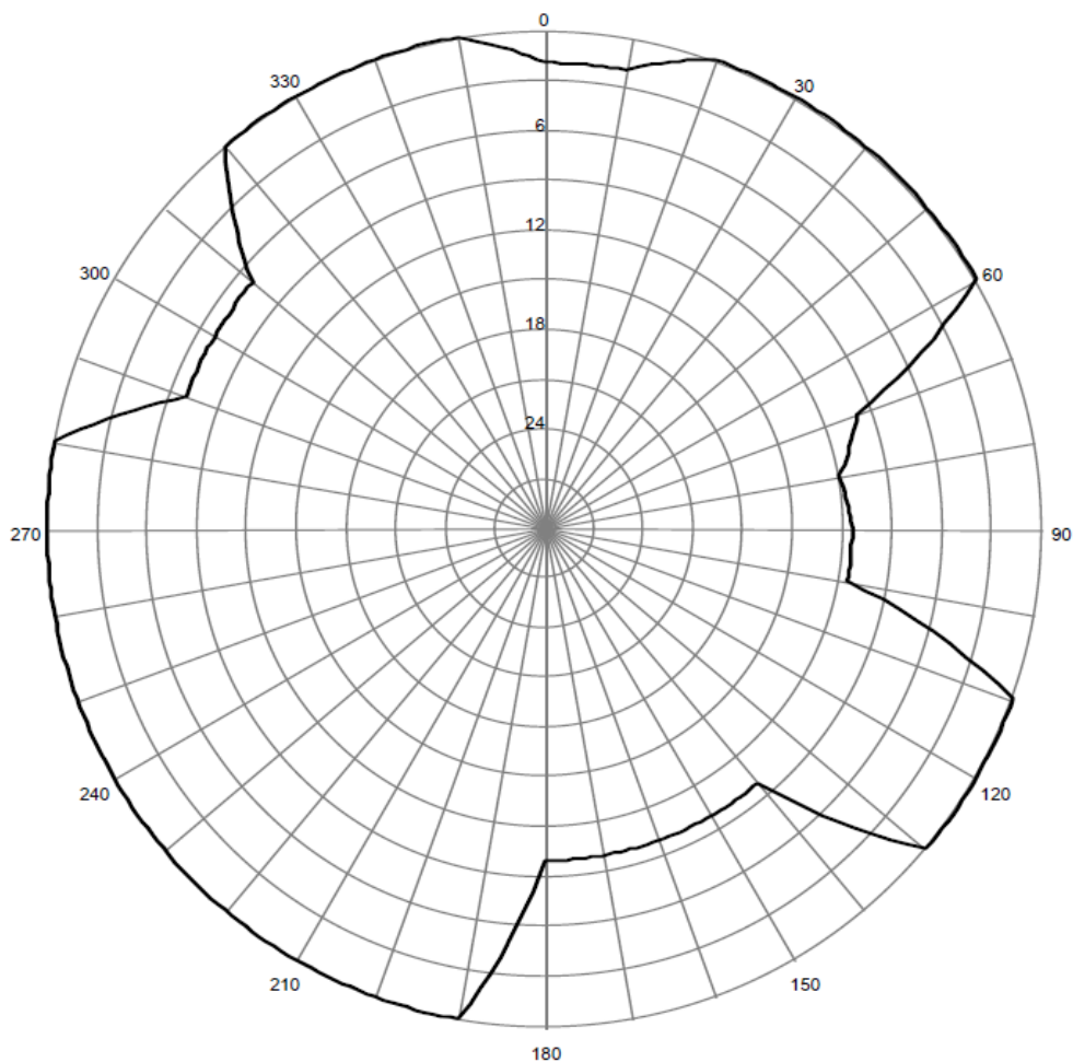
Pozioma charakterystyka promieniowania anteny stacji Przemysł 93,20 MHz
