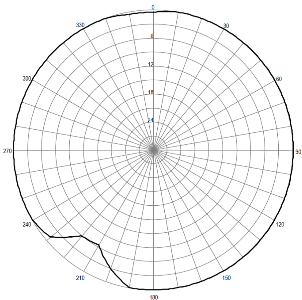
Pozioma charakterystyka promieniowania anteny stacji Sokółka 91,30 MHz
