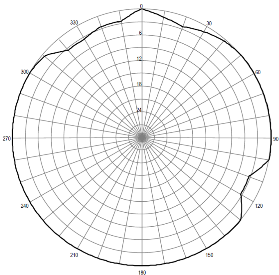
Pozioma charakterystyka promieniowania anteny stacji Siemiatycze 92,50 MHz
