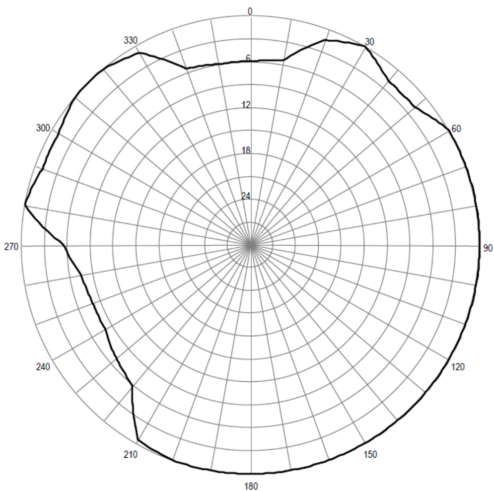
Pozioma charakterystyka promieniowania anteny stacji Bielsk Podlaski 98,70 MHz
