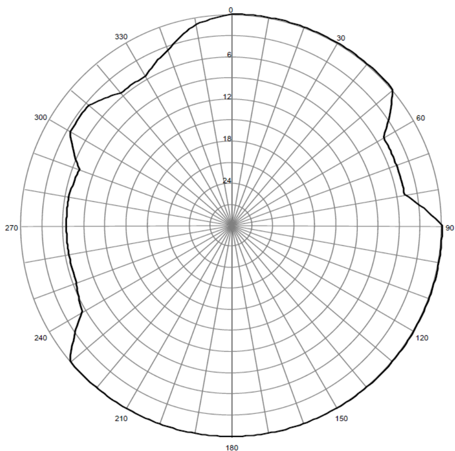
Pozioma charakterystyka promieniowania anteny stacji Białystok 102,70 MHz
