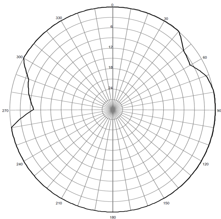
Pozioma charakterystyka promieniowania anteny stacji Białystok 97,50 MHz
