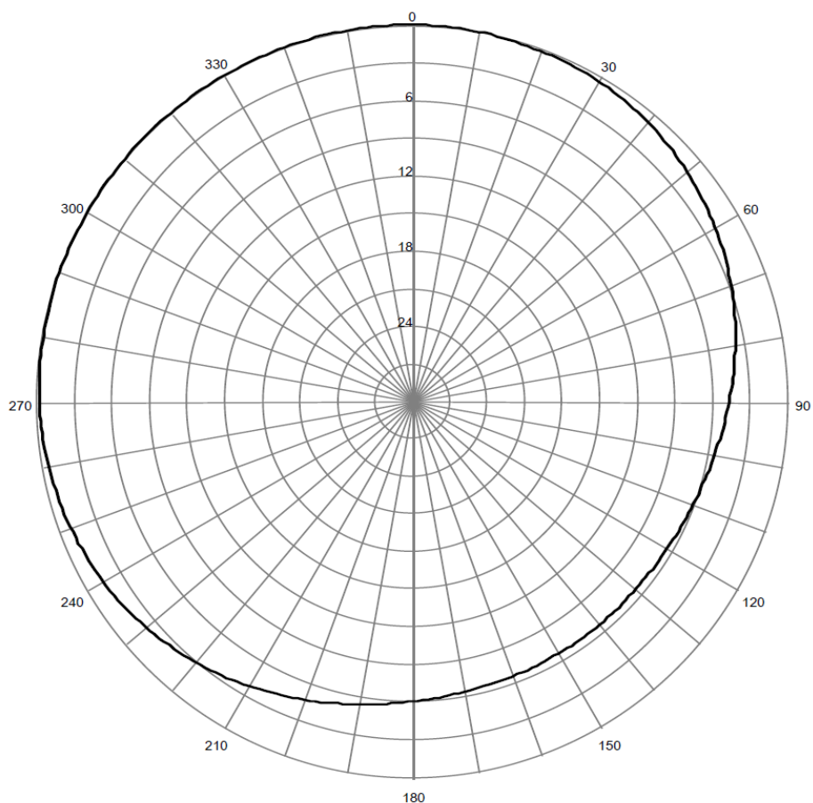
Pozioma charakterystyka promieniowania anteny stacji Łomża 97,50 MHz
