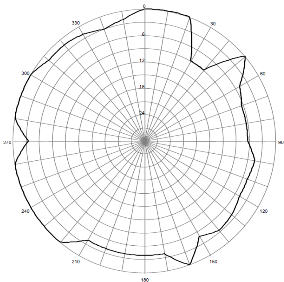
Pozioma charakterystyka promieniowania anteny stacji Łosiów 97,10 MHz
