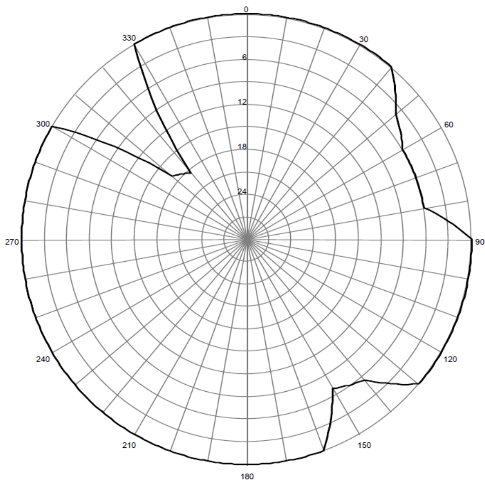
Pozioma charakterystyka promieniowania anteny stacji Wysoka Góra Św. Anny 93,90 MHz
