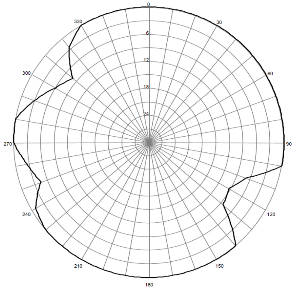
Pozioma charakterystyka promieniowania anteny stacji Opole 99,10 MHz
