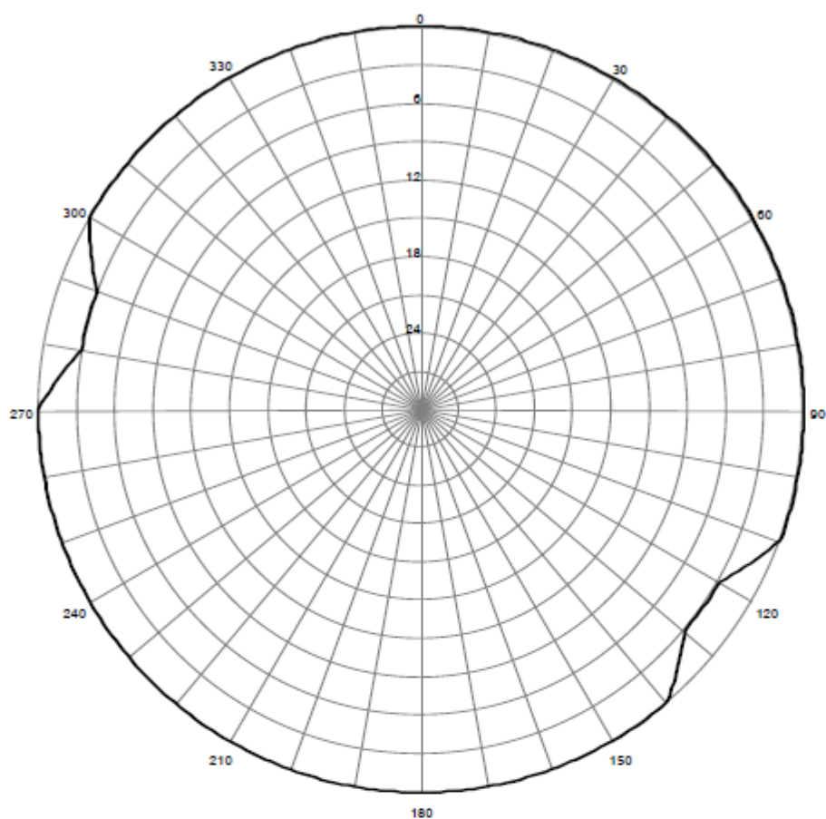
Pozioma charakterystyka promieniowania anteny stacji Poznań 105,40 MHz
