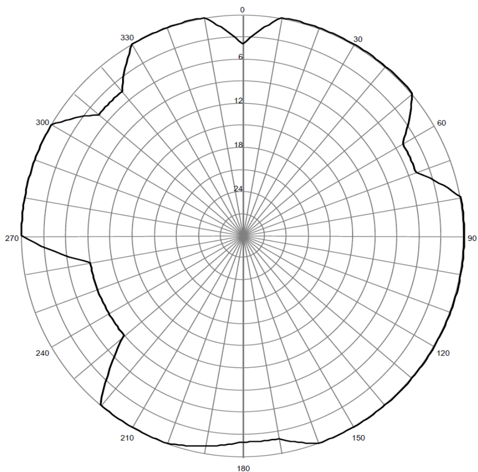
Pozioma charakterystyka promieniowania anteny stacji Białystok 87,70 MHz
